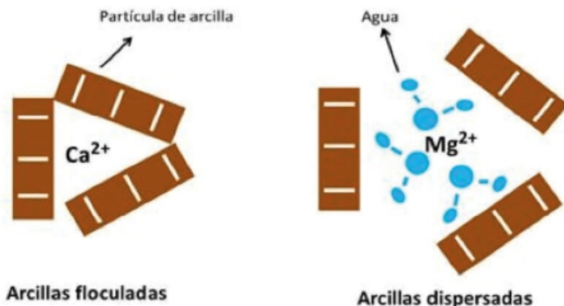
Figura 3. La dispersión en el suelo es causada principalmente por iones altamente hidratados, tales con Na y Mg, atraídos a la superficie de las partículas de arcilla. La adición de calcio soluble puede superar los efectos de la dispersión de iones Na y Mg y ayudar a promover la floculación y desarrollo de una mejor estructura del suelo
